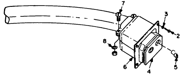
CABLE W1
